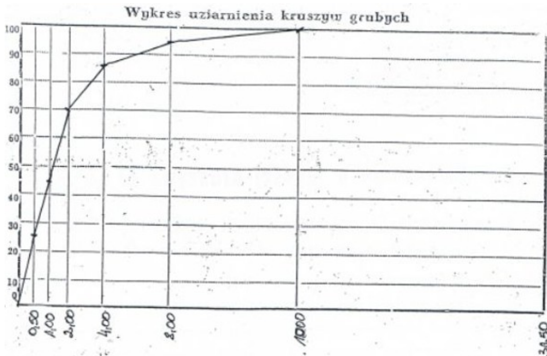
Rysunek 3. Krzywa uziarnienia – mieszanka wbudowana w alejki parkowe jako zamiennik nawierzchni Hanse Grand
